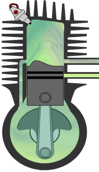
2 zamanlı motor
